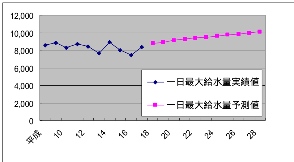
図1 水需要予測
