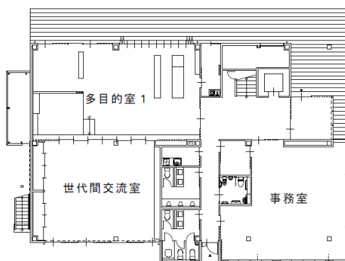
1 階平面図
