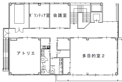
2 階平面図
