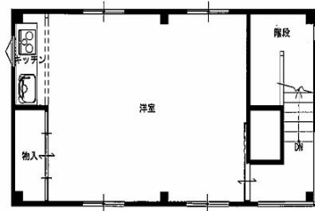
3階 平面図 S:1/100
