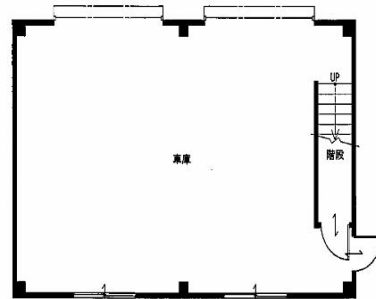
1階 平面図 S:1/100
