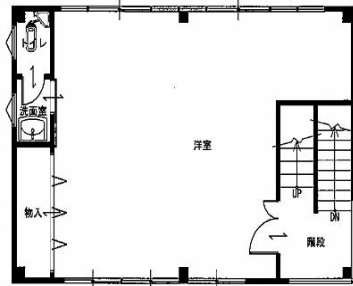
2階 平面図 S:1/100
