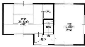
2階 平面図 S:1/50
