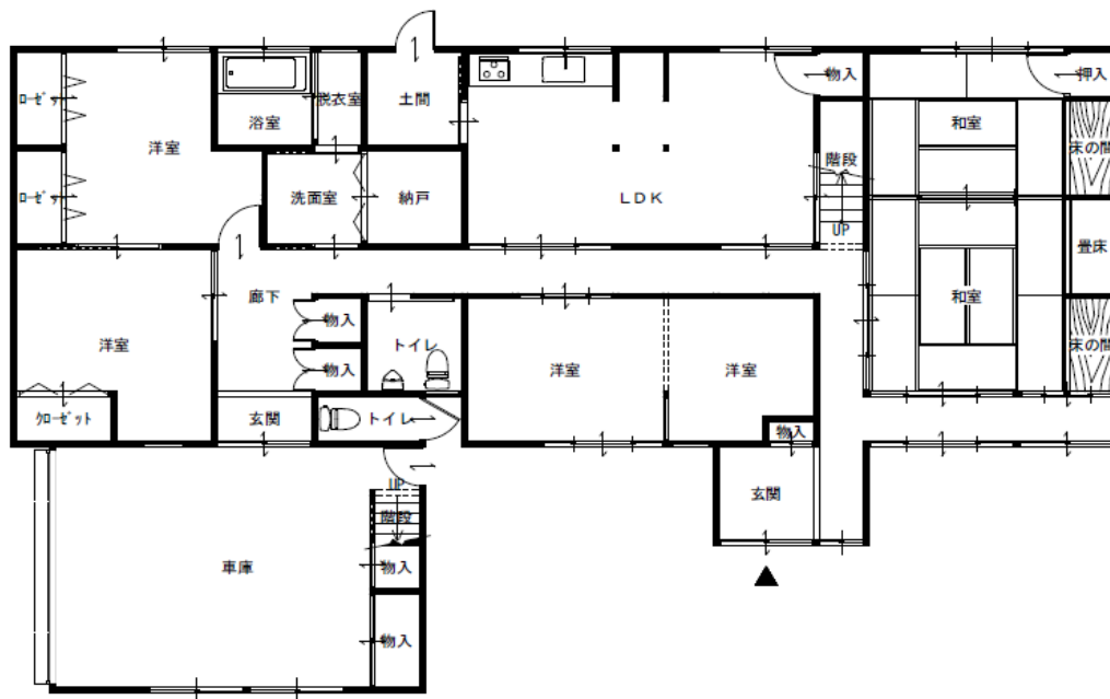
1階 平面図 S:1/80
